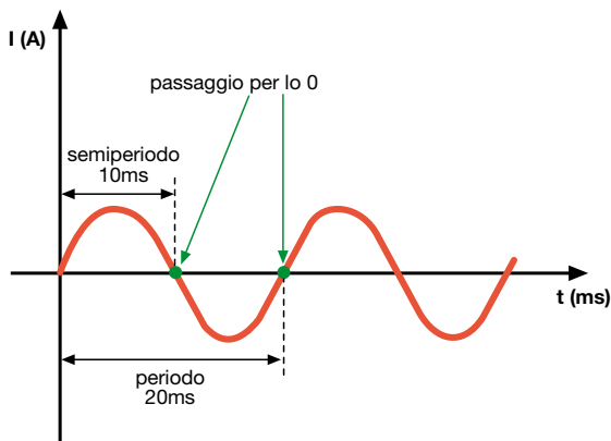
Figura 7 Corrente alternata
