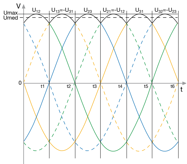
Le linee intere rappresentano l'andamento delle tre sinusoidi delle tensioni concatenate ( U_{12} ; U_{23} ; U_{31} ), mentre le linee tratteggiate le sinusoidi relative alle stesse tensioni ma invertite ( U_{13} = -U_{31} ; U_{21} = -U_{12} ; U_{32} = -U_{23} ).
