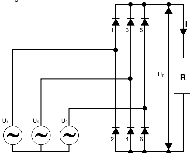
Nello schema si possono distinguere i tre diodi di andata (1,3,5) con i catodi connessi in comune e tre diodi di ritorno (2,4,6) che hanno invece gli anodi connessi in comune.
