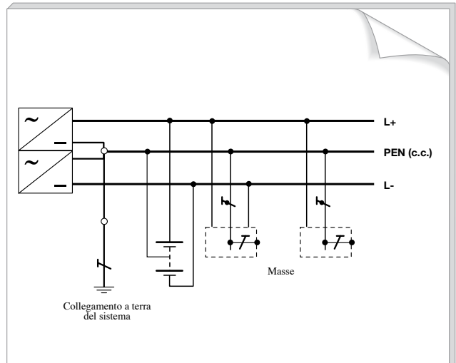
Figura 23 Sistema di distribuzione TN-C in corrente continua con il punto medio dell'alimentazione connesso a terra
